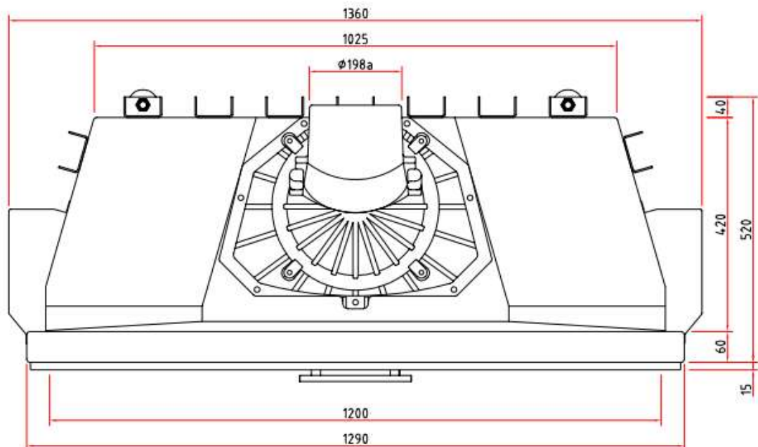
Draufsicht M 1:10
