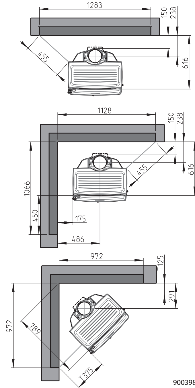
Innfelt brannmur
