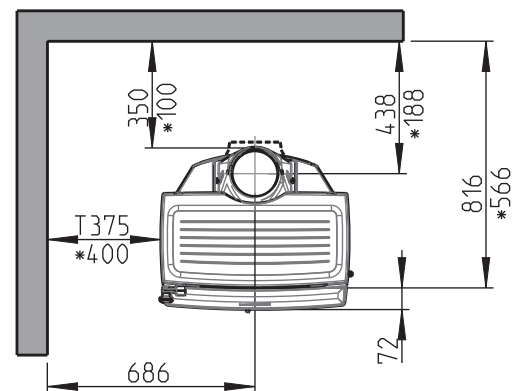
Min. avstand til brennbar vegg
