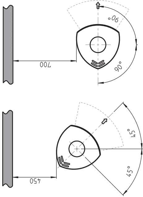
Min. avstånd till brännbar vägg med vridbar pelare
