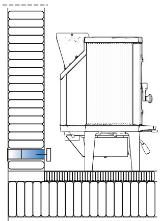
Kuva. 7d Ulkoseinän läpi tulisijan viereen
