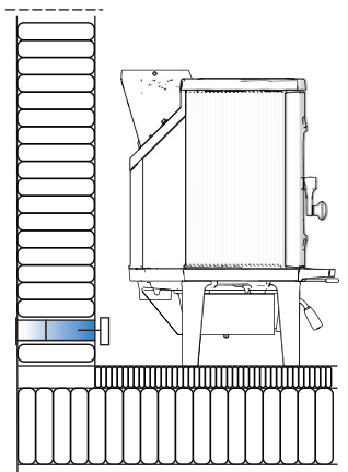
Fig. 7d Indirekte gjennom yttervegg
