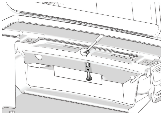
Fig. 21c Udskiftning af ventil
