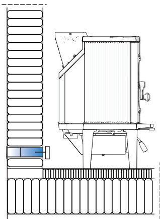
Fig. 7d Indirekte genom yttrevägg
