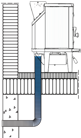
Fig 7c. Gennem gulv og kælder
