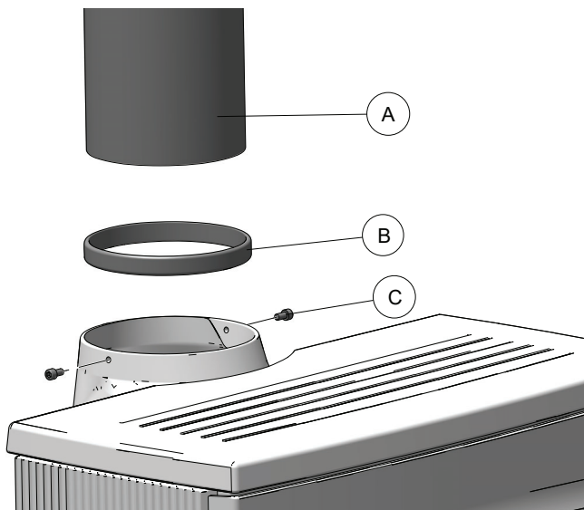
Fig. 6 Montere røgrør
