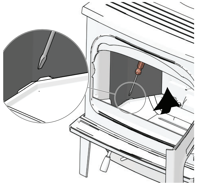
Fig. 18a Utskifting av sidebrennplatene
