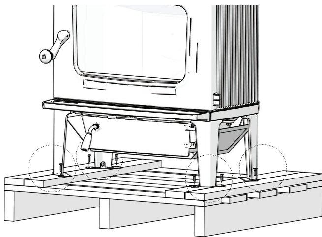
Kuva. 2 Kamiinan irrottaminen kuormalavasta
