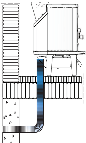
Fig. 7c Genom golv och källare
