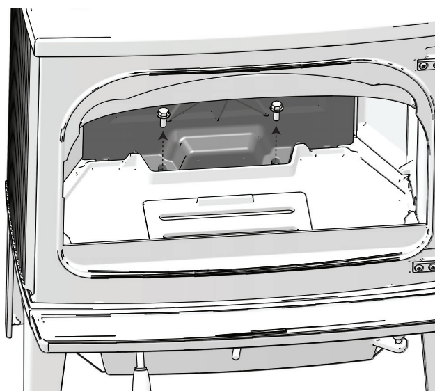
Fig. 19a Byta av bakre eldstadsbeklädnad
