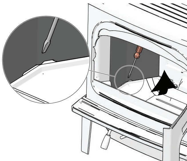
Fig. 18a Udskiftning af side brændepladene
