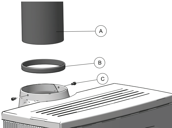
Kuva. 6 Savuputken kiinnittäminen
