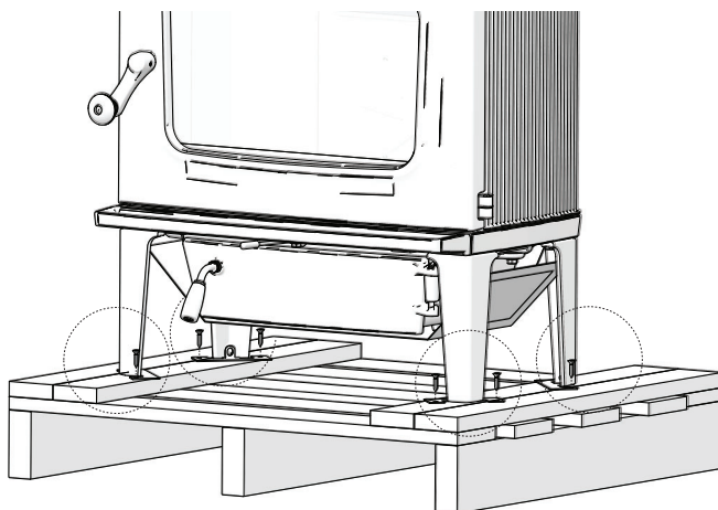
Fig. 2 Släpp från pall
