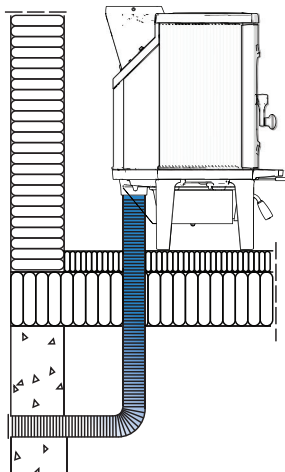
Kuva. 7c Lattian ja kellartilan läpi
