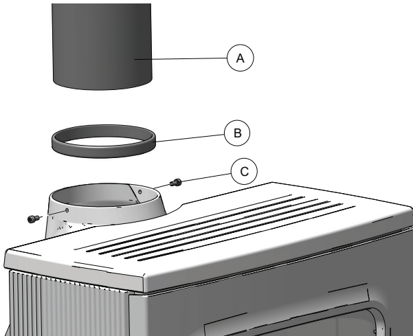
Fig. 6 Montere røykrør
