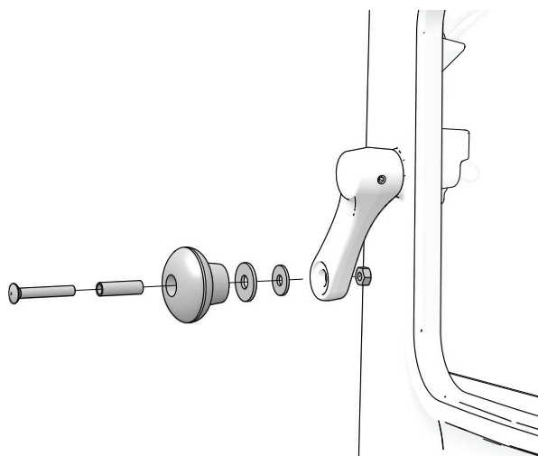
Fig. 3 Handtag montering
