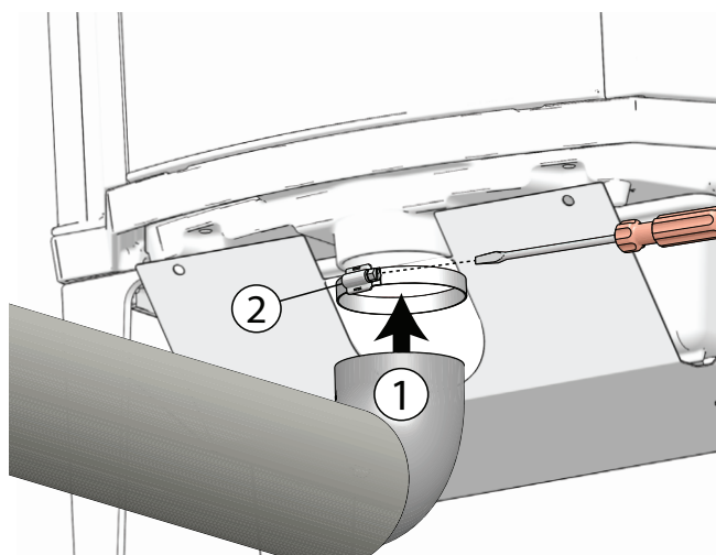
Fig. 8b Montering af udeluftstilførsel
