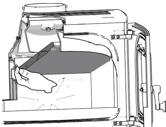
Fig. 16b Fjernelse af røgvenderplade
