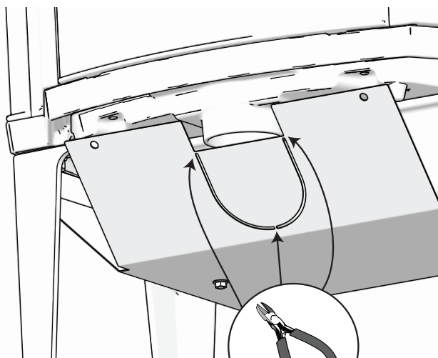
Fig. 8a Montering av frislutstillförel
