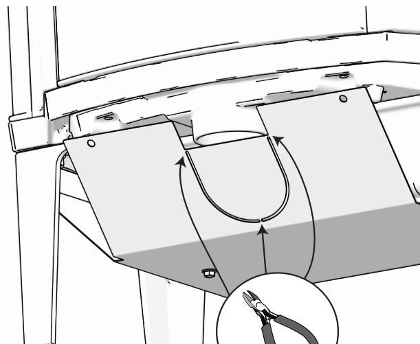
Fig. 8 Montering af udeluftstilførsel
