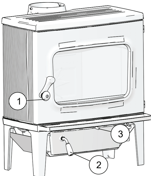
Fig. 10 Betjeningsmuligheter på Jøtul F 405
