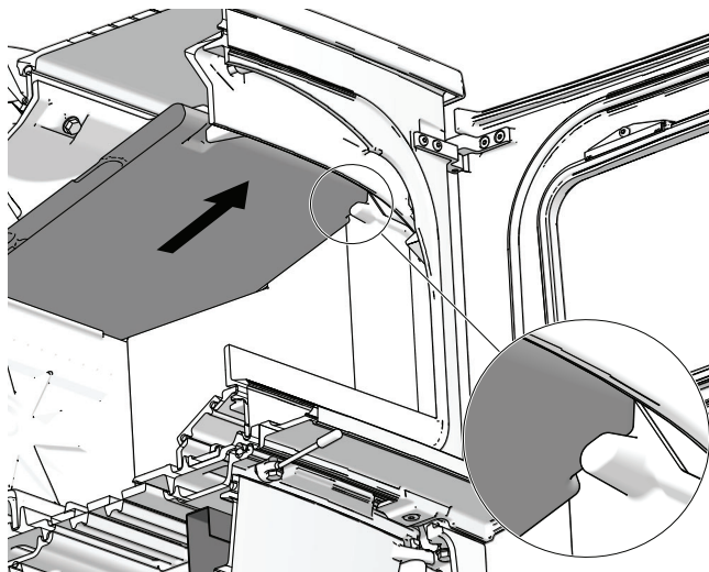
Fig. 16a Lossa rökhylla
