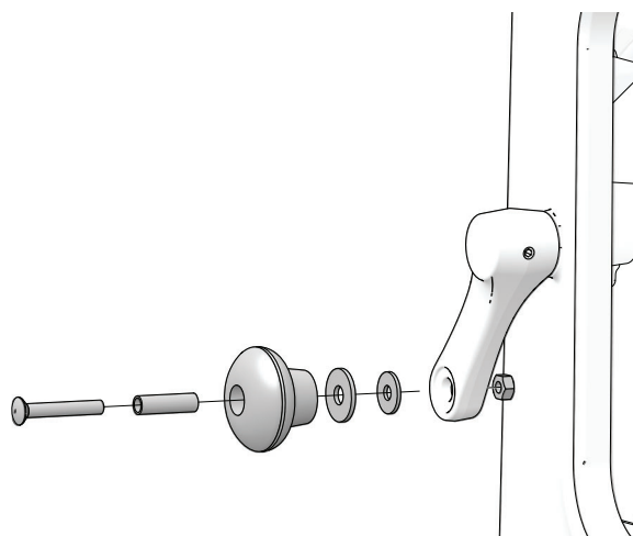
Fig. 3 Feste av dørhåndtak
