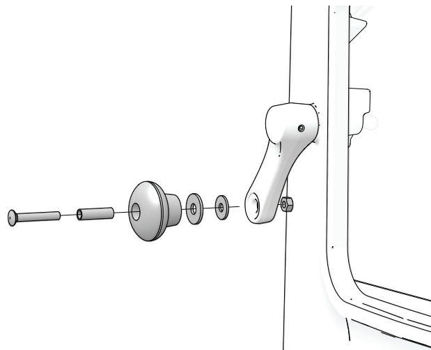
Kuva. 3 Asennus kahvaan
