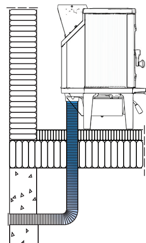
Fig. 7c Gjennom gulv og kjeller
