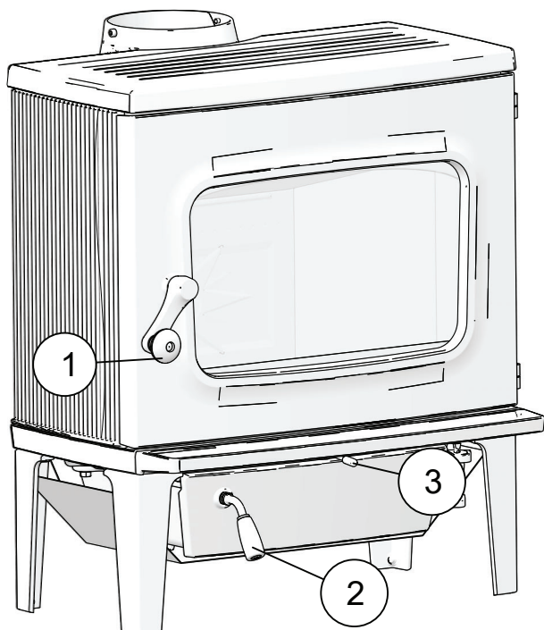
Fig. 10 Inställningsmöjligheter på Jøtul F 405
