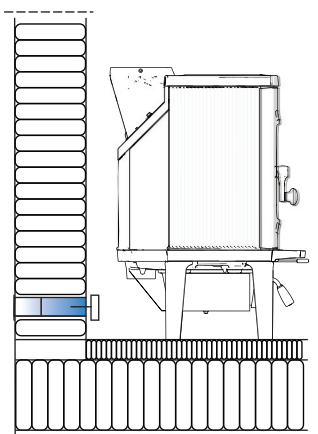
Fig 7d. Indirekte gennem ydervæg
