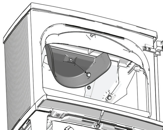
Fig. 17 Udskiftning af ledeplade
