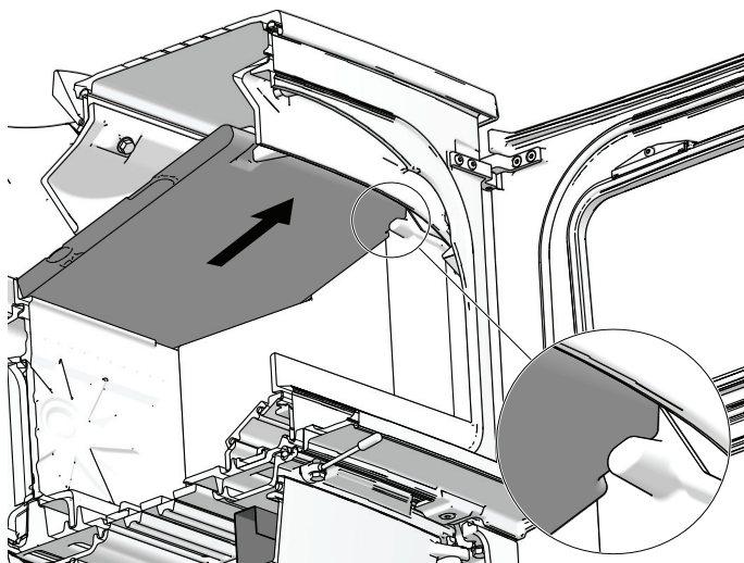
Fig. 16a Løsne hvelv
