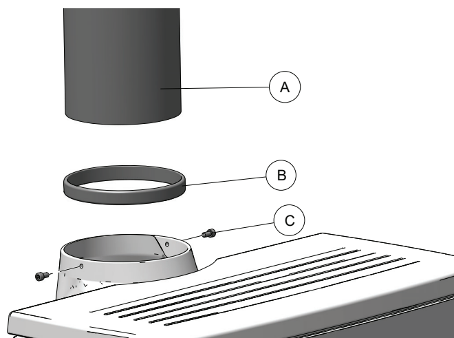
Fig. 6 Montering av rökrör
